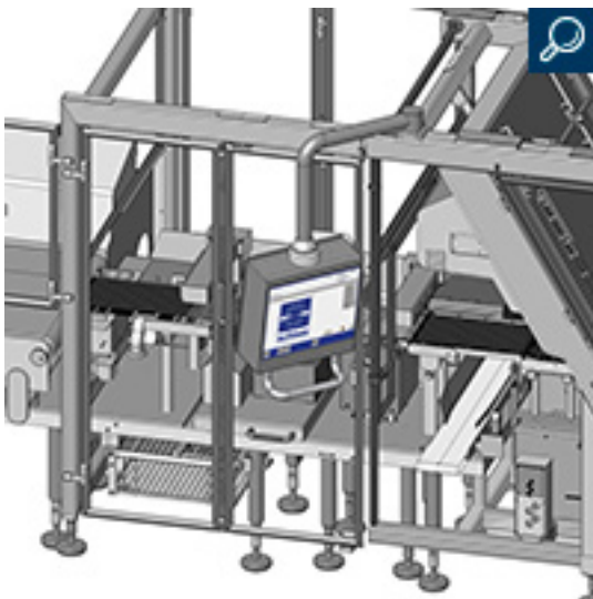
Rohschinken-Schneidelinie Interleaver
